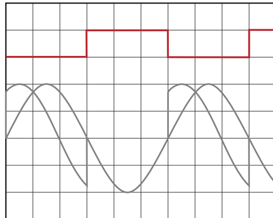
Fig. 1: PSK-signal: Ph0 = 0, Ph1 = 70 degr.
